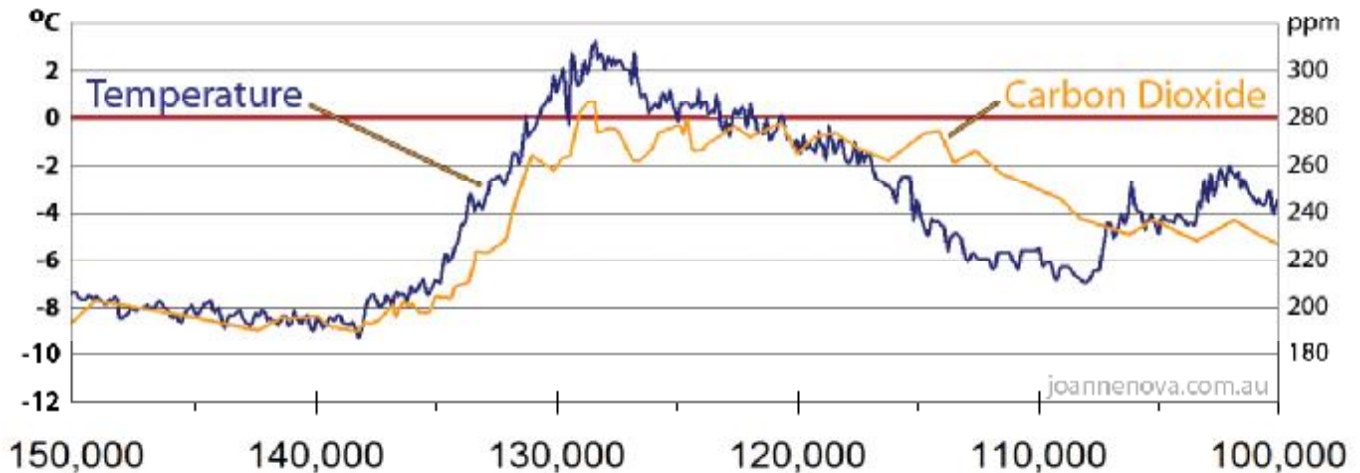
Vostok Ice Cores 150,000 - 100,000 years ago
